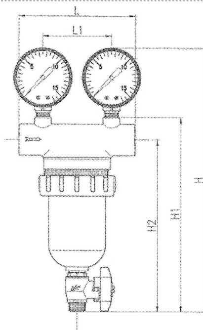
Abb. 1: Abmessungen Schutzfilter
